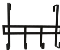
FA-BK5827 Door hooks
